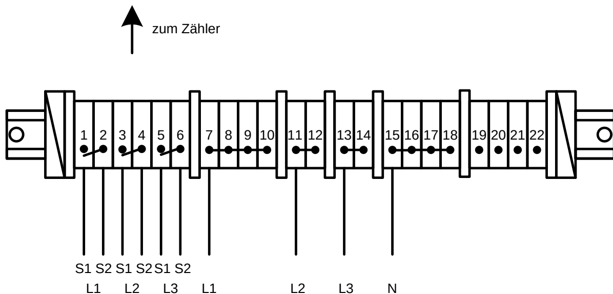
A 1.02 Klemmenleiste für den Einsatz auf Wechseltafeln sowie im Zählerfeld
